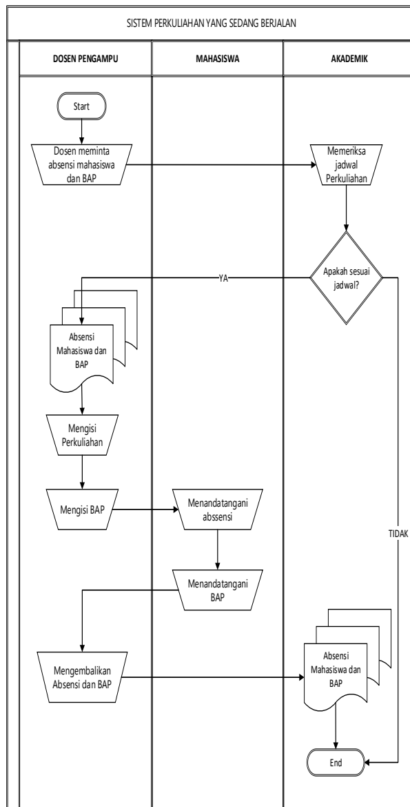
Gambar 4. Flowmap Perkuliahan yang Sedang Berjalan
