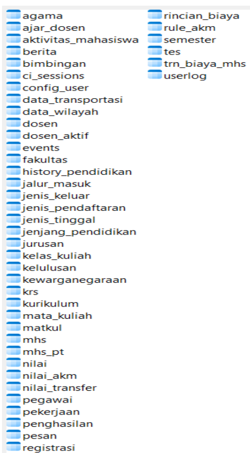
Gambar 8. Database SIAKAD STMIK Lombok
