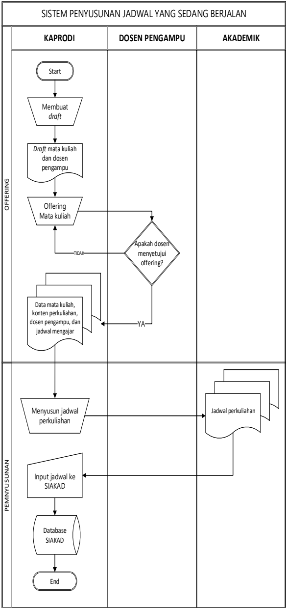
Gambar 2. Flowmap Penyusunan Jadwal yang Sedang Berjalan
