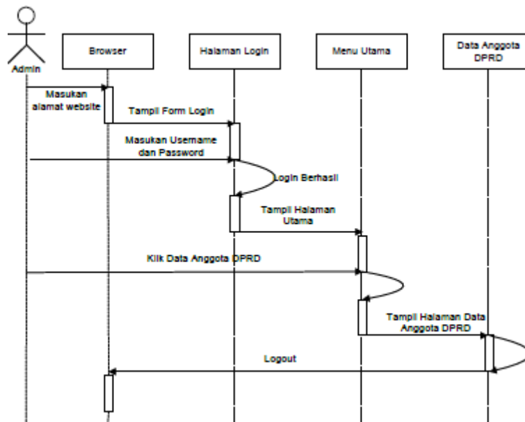
Gambar 5. Sequence Diagram Admin Melihat Data Anggota DPRD
