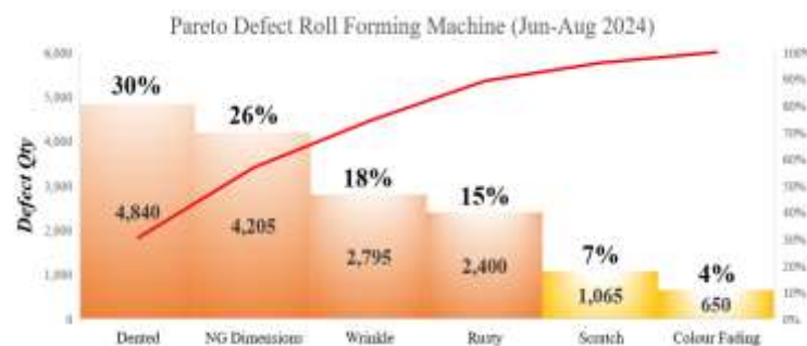
Gambar 2. Diagram pareto defect pada mesin roll forming
