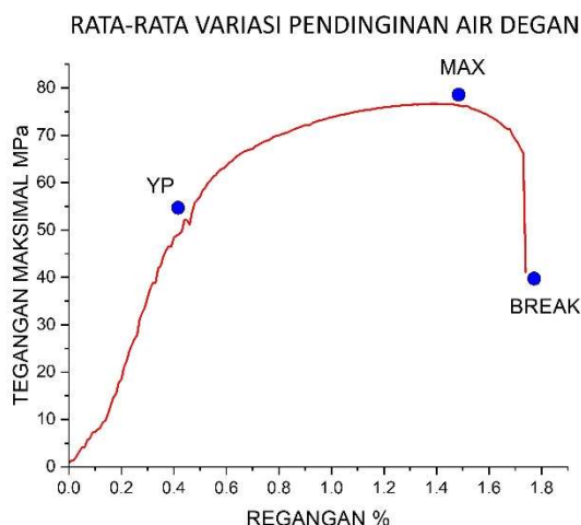
Gambar 5. Grafik rata-rata pengujian spisemen variasi degan
