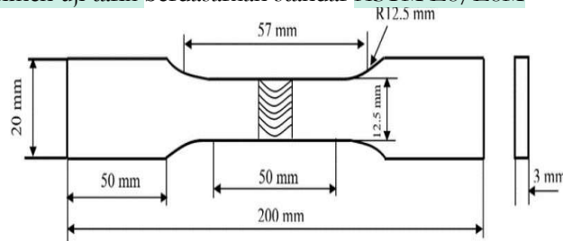
Gambar 1 Spesimen uji tarik ASTM/E8/E8M-09
