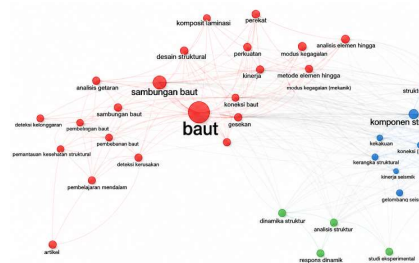
gambar 4. jaringan co-occurrence sambungan baut dan las baja
