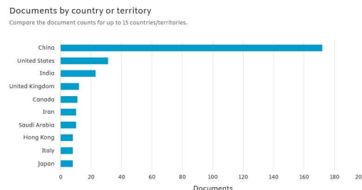
gambar 2. Jumlah publikasi berdasarkan negara
