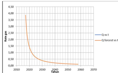
Gambar 4. Prediksi Produksi Menggunakan Decline Curve Analysis (DCA)
