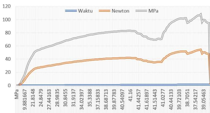
Gambar 4.1 Grafik Hasil Uji Bending
