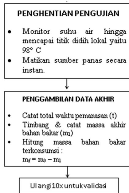
Gambar 2. Skema eksperimen.
