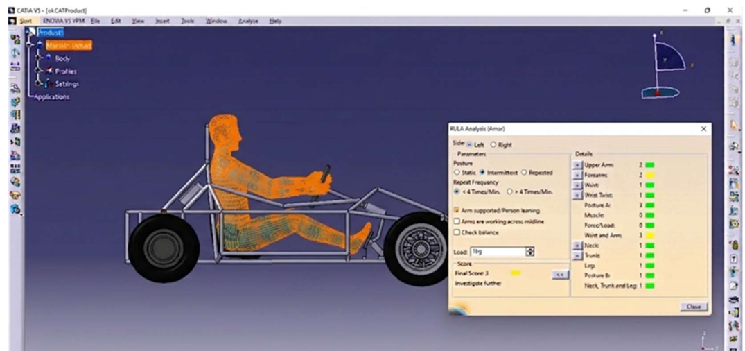
Gambar 3. Pemodelan Postur Pengemudi pada Mobil Listrik 2 kW BARATA Menggunakan CATIA V5.
