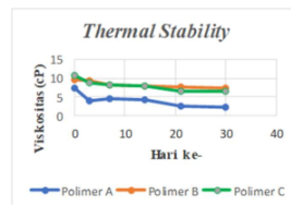
Gambar 3. Perubahan viskositas polimer selama pengujian stabilitas termal pada temperatur 60°C.
