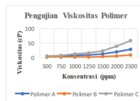
Gambar 3. Hubungan konsentrasi polimer terhadap viskositas larutan.
