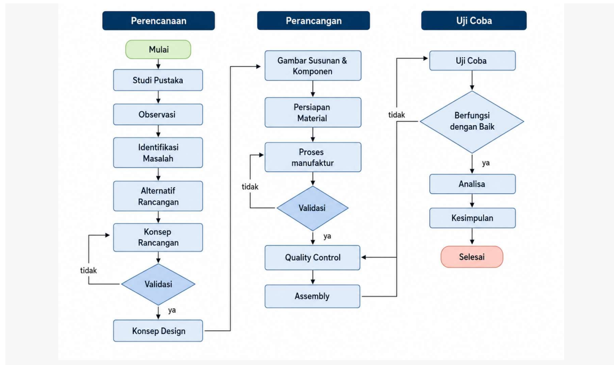
Gambar 1. Diagram alir metodologi penelitian (tempel manual dari sumber PDF/laporan).
