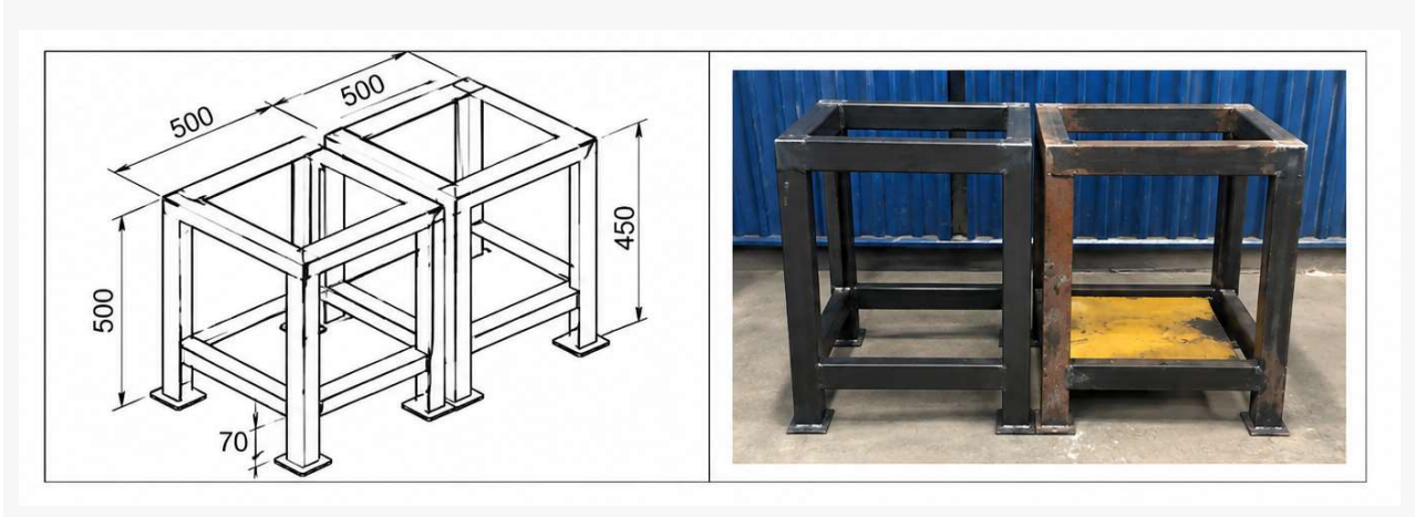
Gambar 8. Rangka mesin dan proses manufaktur rangka
