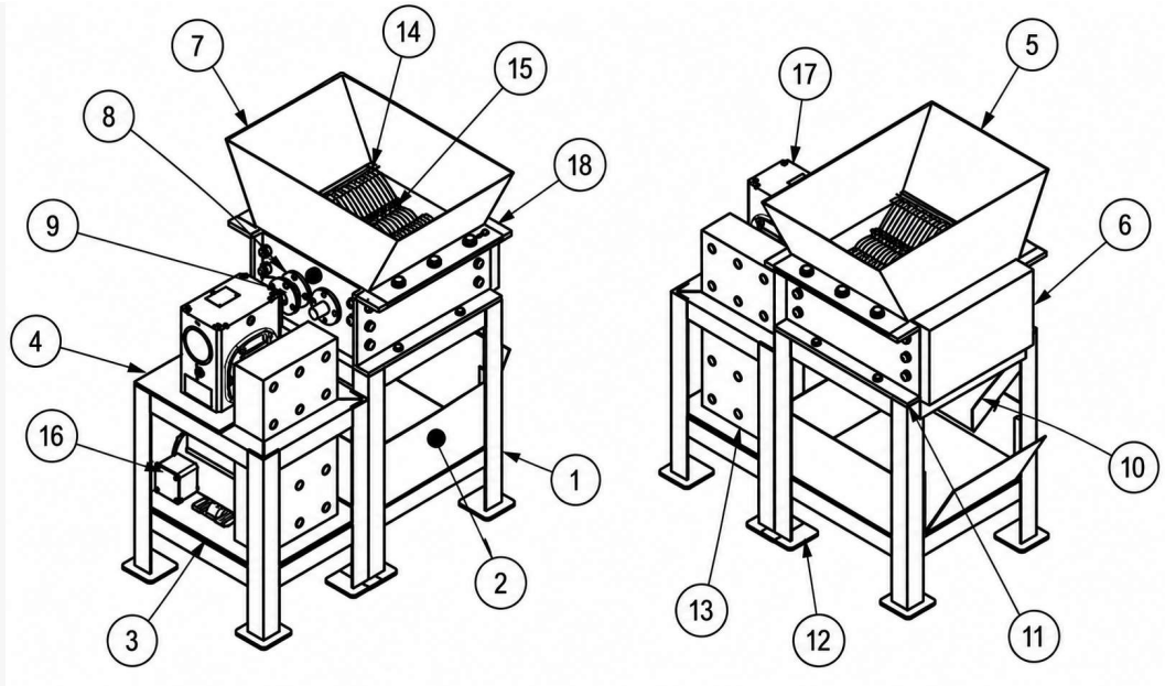
Gambar 2. Rancangan mesin pencacah plastik tipe shredder
