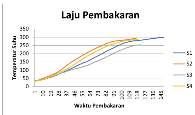
Gambar 4.1 Grafik Hasil Uji Laju Pembakaran
