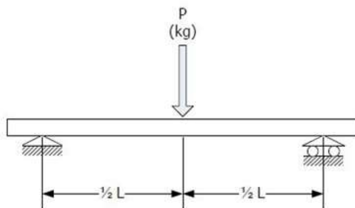
Gambar 2.2 Pembebanan Uji Bending (Sumber: Rajasensor, 2021)
