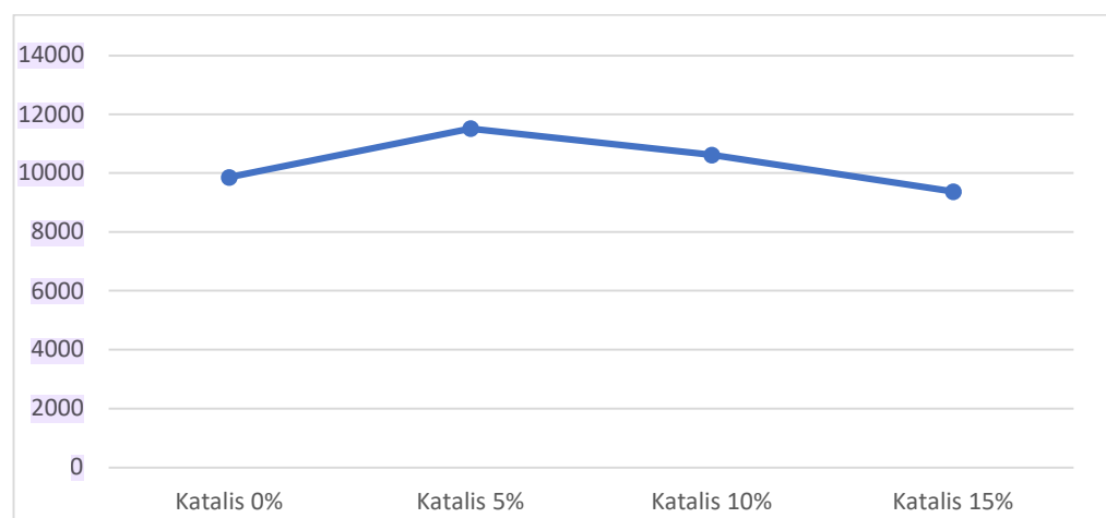
Gambar 1 Grafik Hasil Pengujian Nilai Kalor
