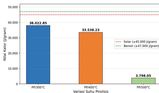
Gambar 4.1 Grafik Nilai Kalor
