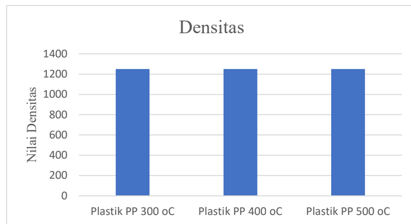
Gambar 4. 2 Grafik Densitas
