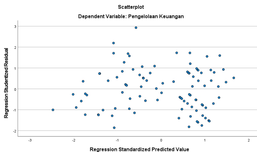
Gambar 1. Uji Heteroskedastisitas
