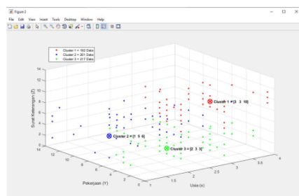
Gambar 3. Grafik Cluster
