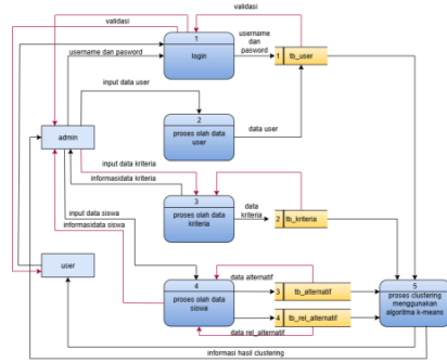
Gambar 2. DFD Level 1
