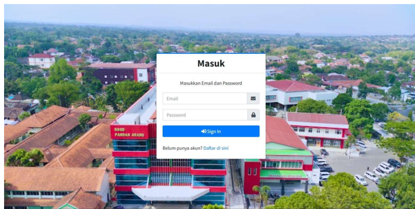
Gambar 5. Halaman Login
