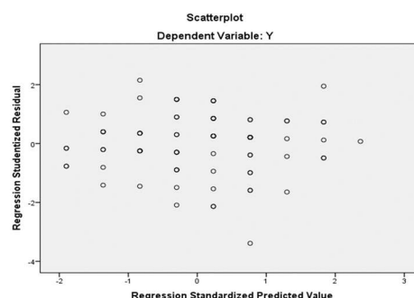
Gambar 8. Uji Heteroskedastisitas
