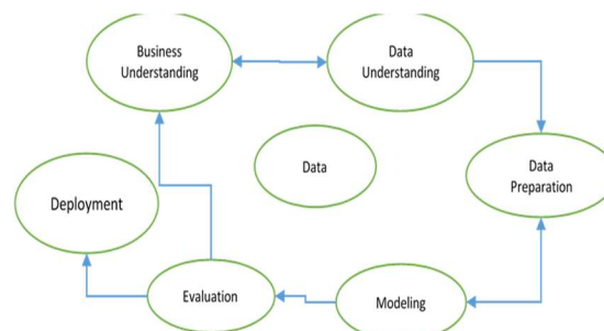
Gambar 1. Tahapan CRISP-DM
