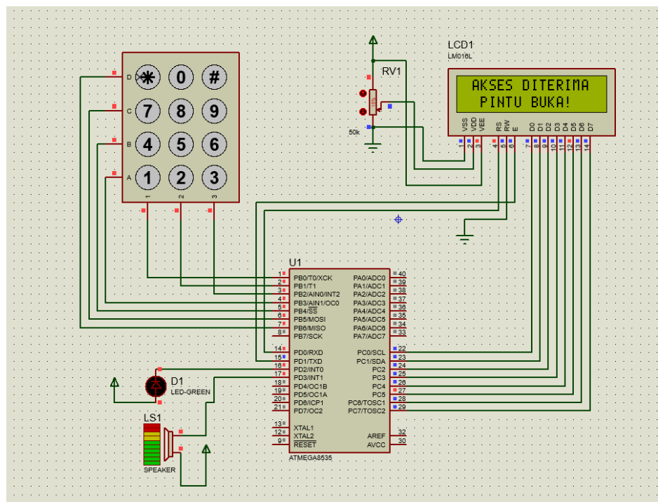
Gambar 4. Hasil pengujian pada proteus
