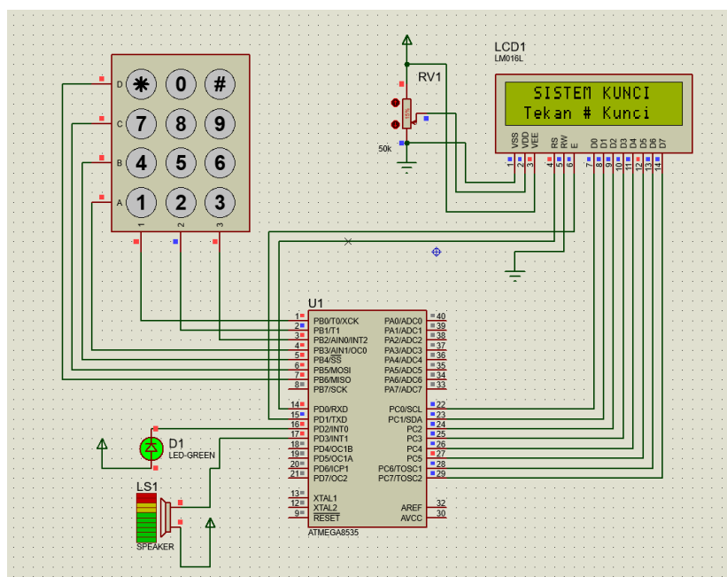
Gambar 1. Skematik Alat
