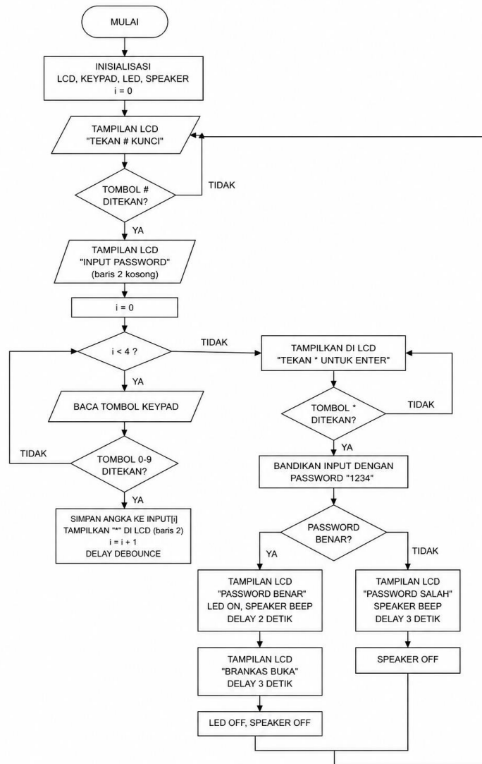
Gambar 3. Alur Sistem
