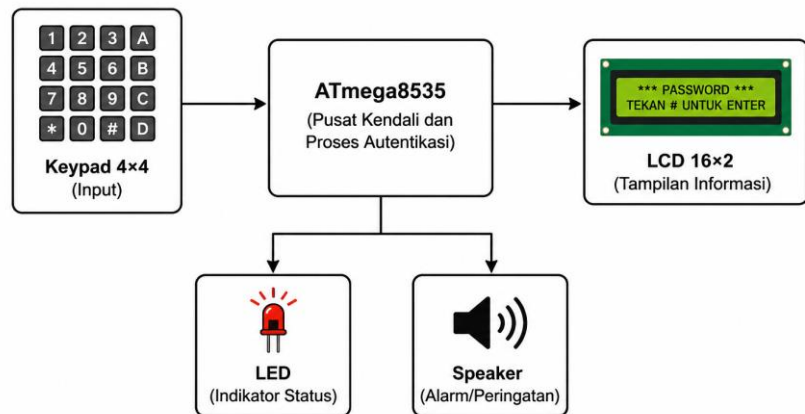
Gambar X. Diagram Blok Sistem Pengunci Brankas Digital Berbasis ATmega8535
