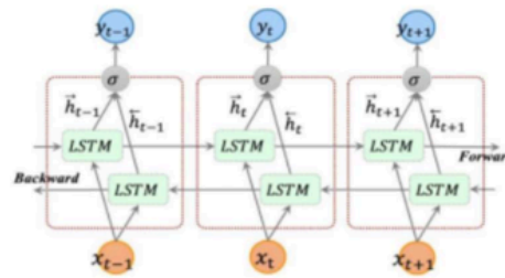
Gambar 1. Arsitektur BiLSTM
