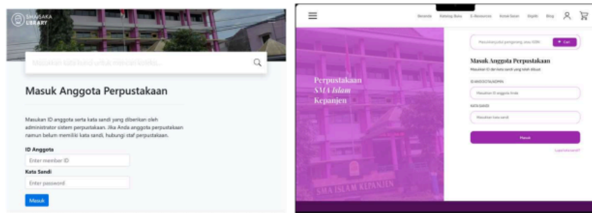
Gambar 3. Halaman login SLiMS sebelum (a) dan sesudah (b) redesain dengan perubahan pada warna dan tata letak.
