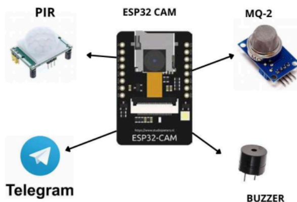
Gambar 2. Perancangan Sistem
