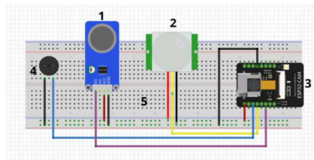
Gambar 3. Rangkaian Seluruh Sistem
